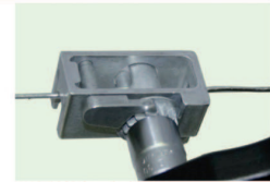
GS*-Drahtspanner
